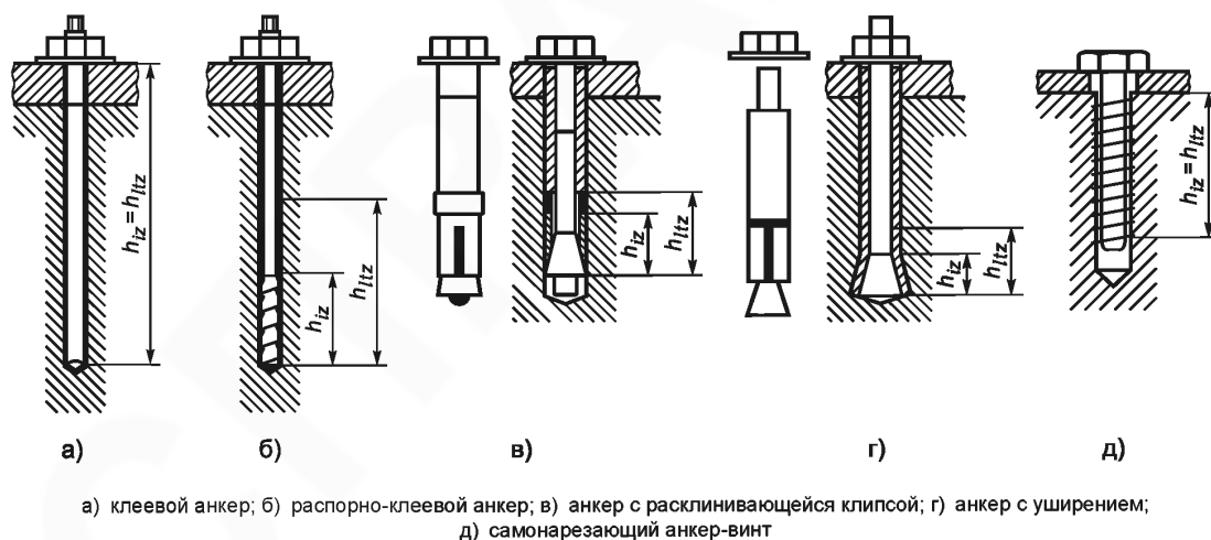
Рисунок 7.4 — Зона эффективного восприятия нагрузки, h_{ltz}
