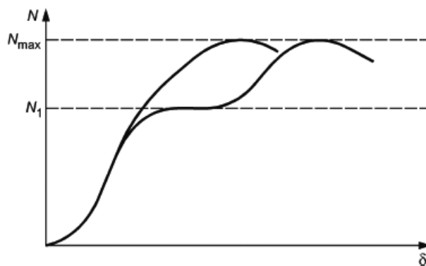
Рисунок 5.1 - График "нагрузка - перемещение" для анкеров КМ
