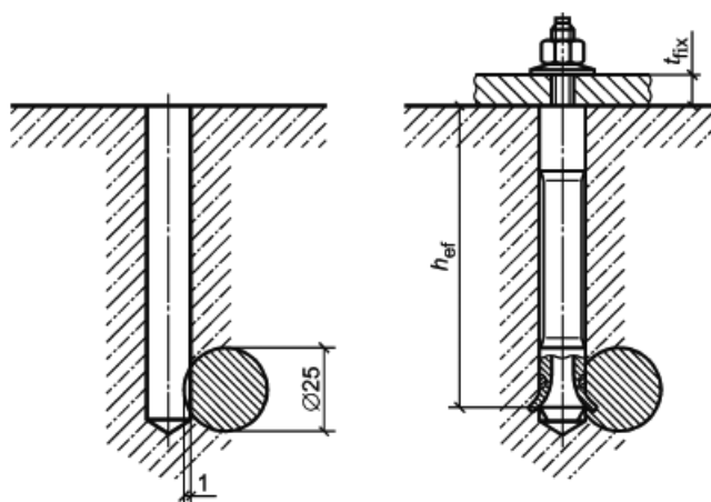
Рисунок 7.2 - Схема испытания анкера при влиянии армирования основания
